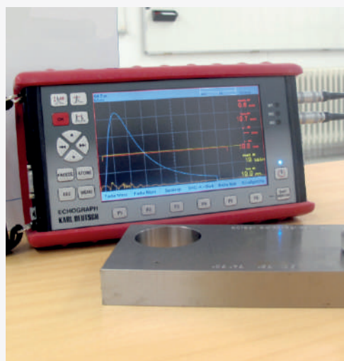
ECHOGRAPH 1095
